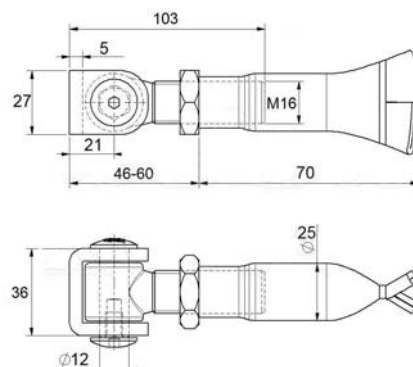
PAX M16 – do zdi s kontramaticí
