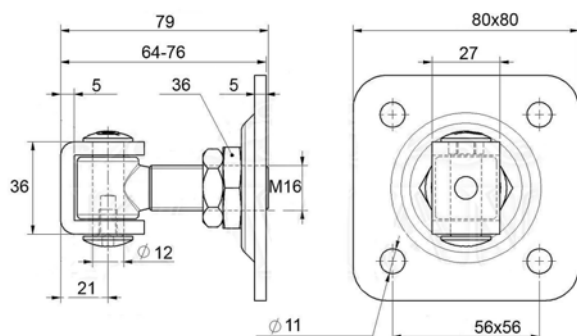
PAZ M16 – regulovatelný s deskou a kontramaticí
