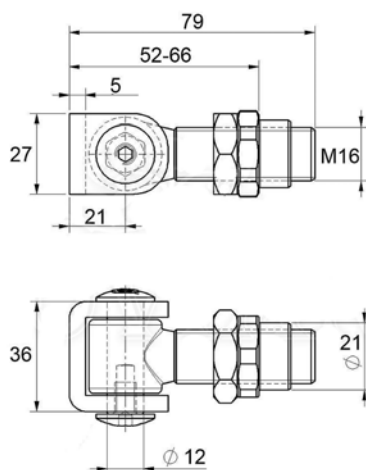
PA M16 – navařovací s kontramaticí
