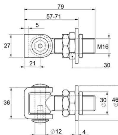
PAR M16 – regulovatelný, navařovací s kontramaticí
